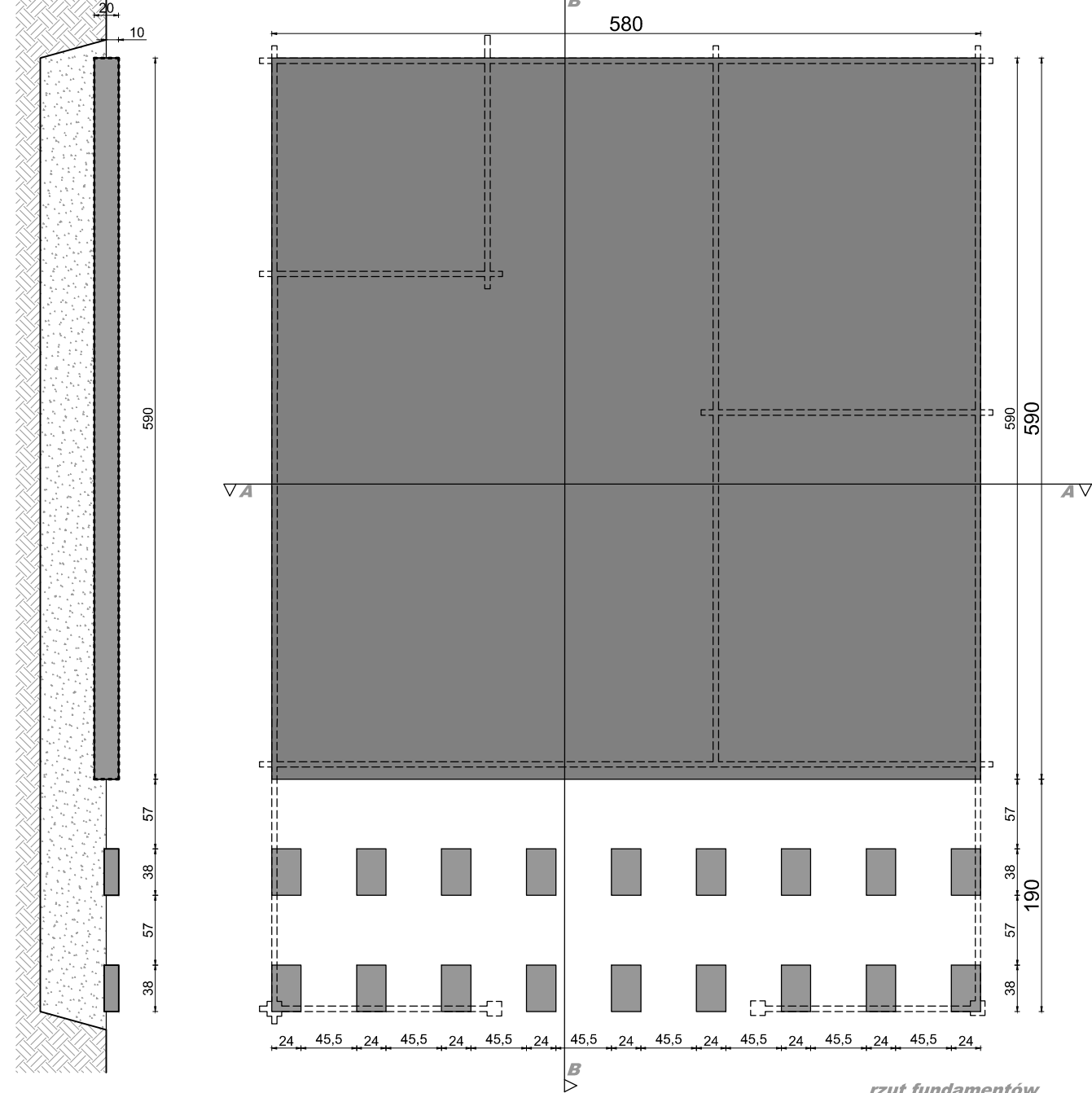
przekrój B-B
