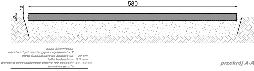
rzut fundamentów
