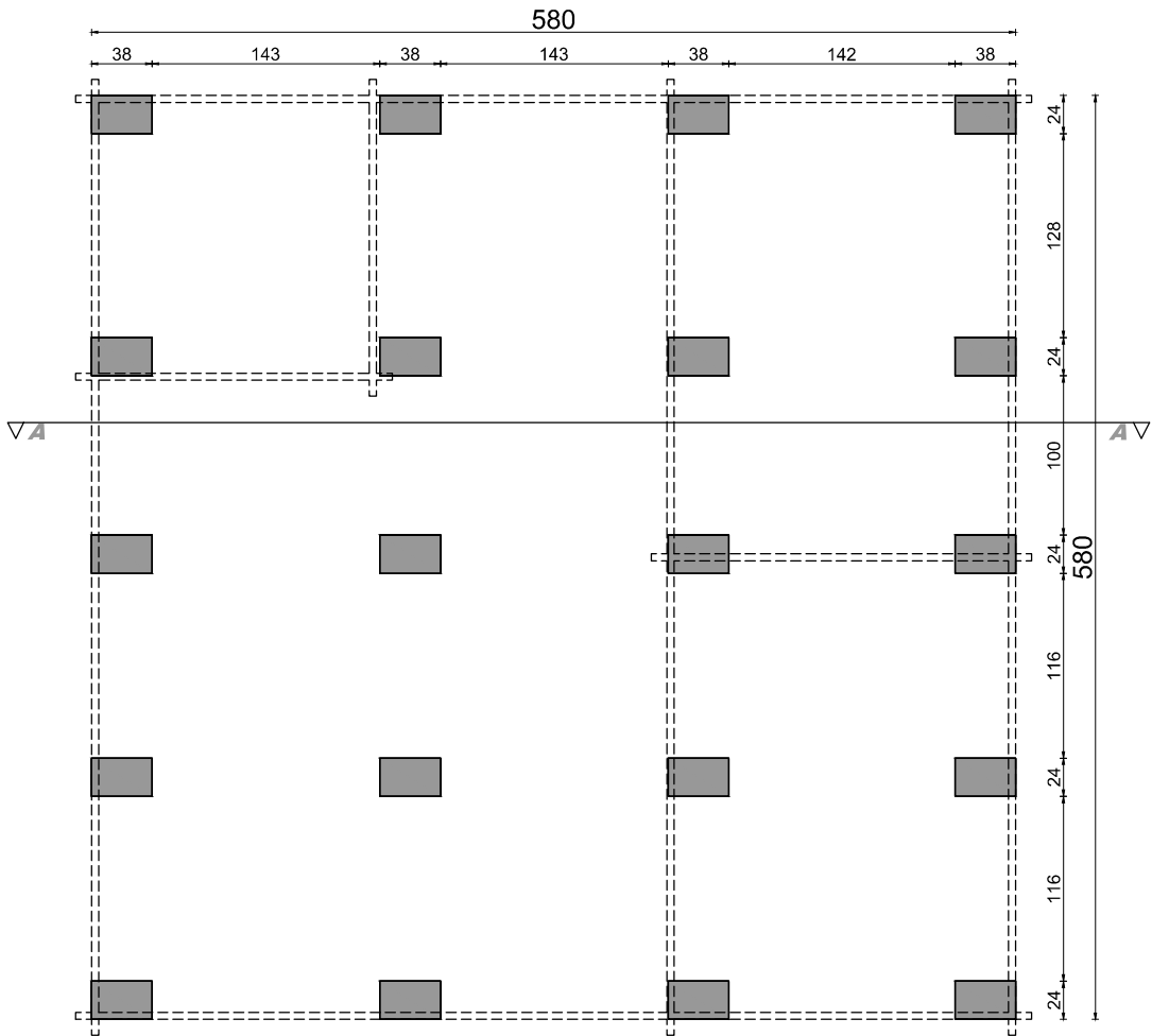
rzut fundamentów
